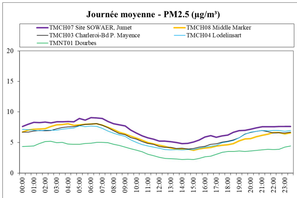
Figure 4.5.2 : PM2.5 – Journée moyenne – (01/01/2024 au 30/06/2024)
