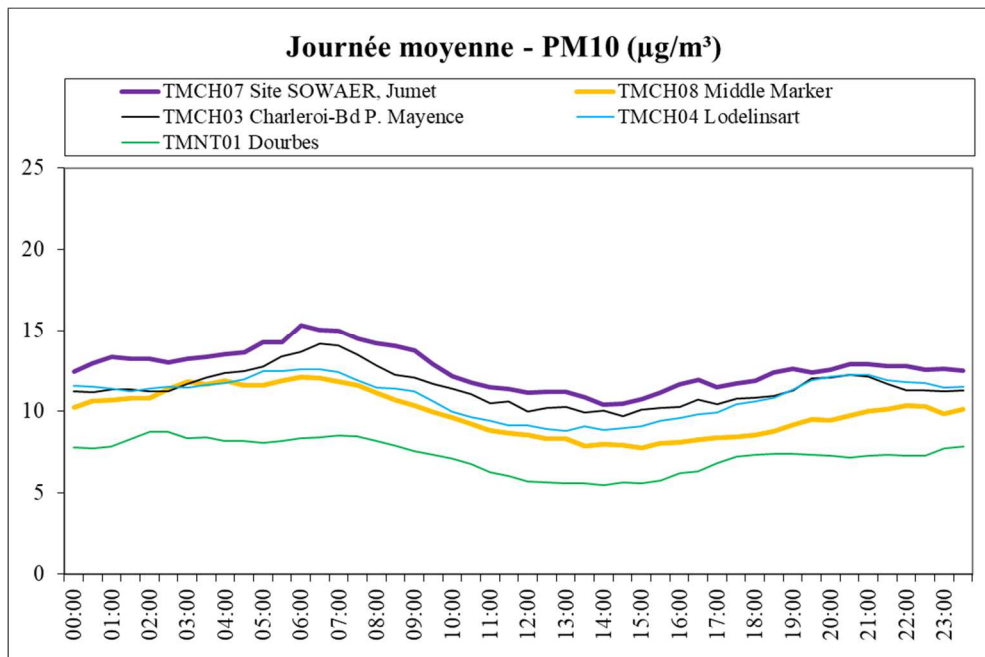
Figure 4.3.2 : PM10 – Journée moyenne – (01/01/2024 au 30/06/2024)
