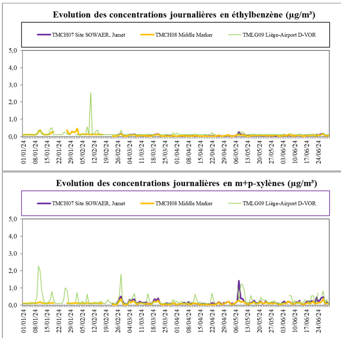
Figure 7.3.1 : BTEX – Evolution des concentrations journalières – (01/01/2024 au 30/06/2024)
