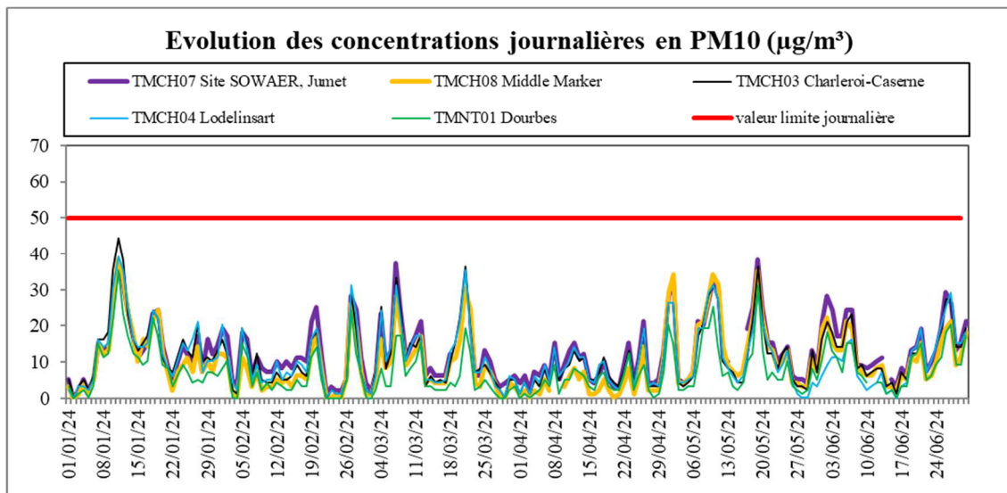
Figure 4.3.1 : PM10 – Evolution des concentrations journalières – (01/01/2024 au 30/06/2024)
