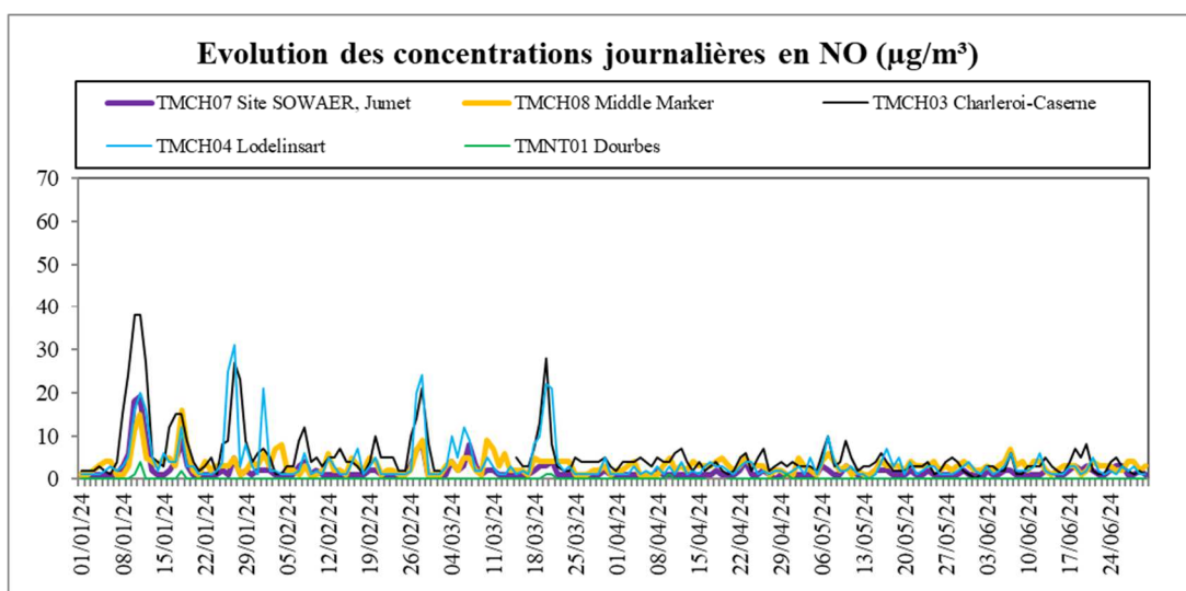
Figure 6.3.1 : Monoxyde d'azote (NO) – Evolution des concentrations journalières – (01/01/2024 au 30/06/2024)
