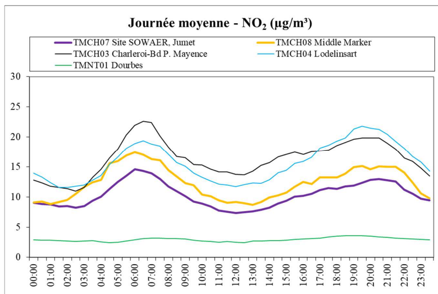
Figure 6.5.2 : Dioxyde d'azote (NO 2 ) – Journée moyenne – (01/01/2024 au 30/06/2024)
