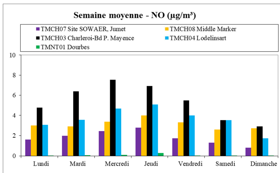
Figure 6.3.3 : Monoxyde d'azote (NO) – Semaine moyenne – (01/01/2024 au 30/06/2024)
