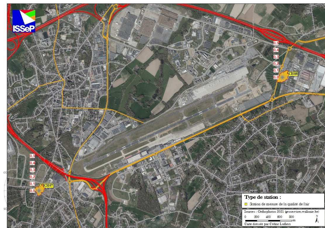
Figure 7.3.4 : Ethylbenzène ( C_6H_5-C_2H_5 ) – Roses de pollution – (01/01/2024 au 30/06/2024)
