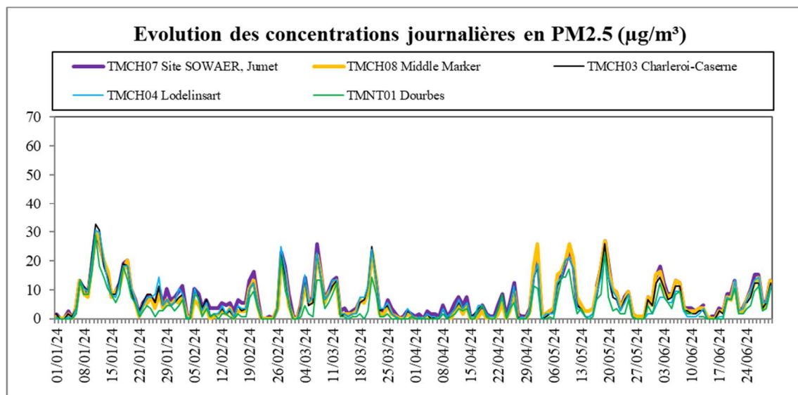
Figure 4.5.1 : PM2.5 – Evolution des concentrations journalières – (01/01/2024 au 30/06/2024)
