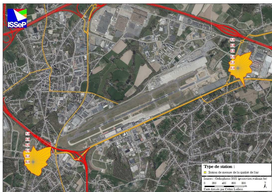
Figure 7.3.3 : Toluène ( C_6H_5-CH_3 ) – Roses de pollution – (01/01/2024 au 30/06/2024)
