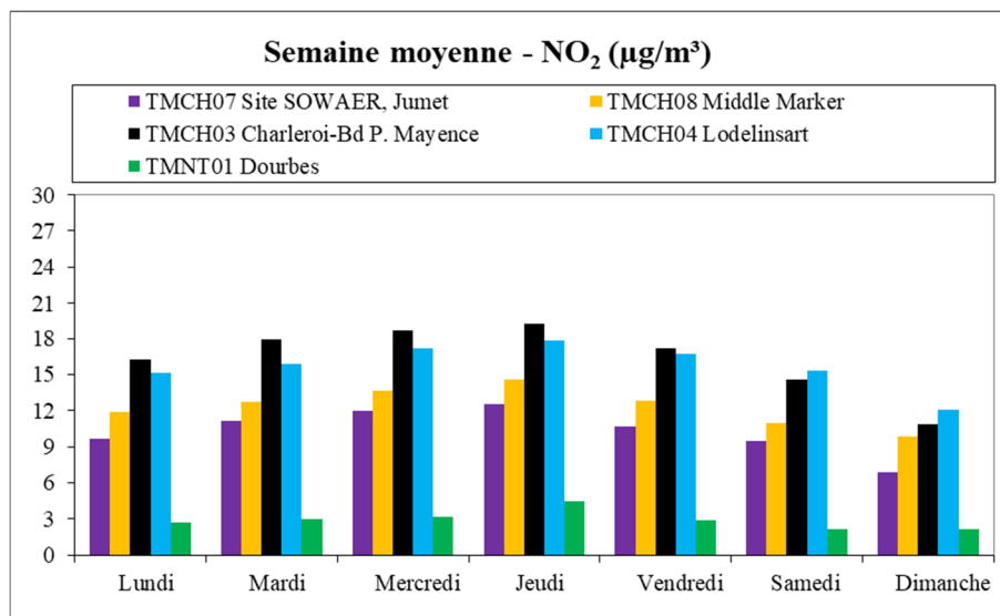
Figure 6.5.3 : Dioxyde d'azote (NO 2 ) – Semaine moyenne – (01/01/2024 au 30/06/2024)
