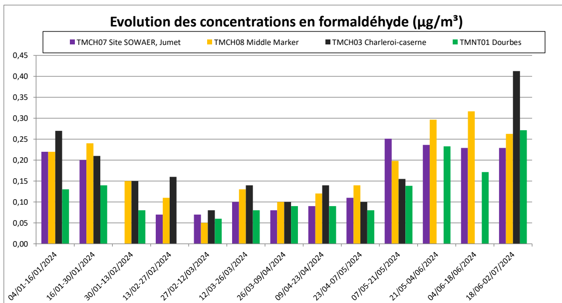
Figure 9.3.1 : Formaldéhyde (CH 2 O) – Evolution des concentrations bimensuelles – (04/01/2024 au 02/07/2024)
