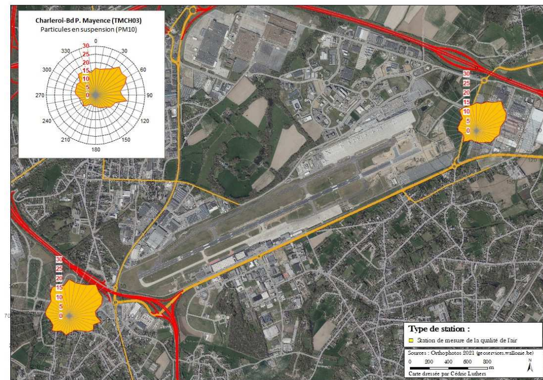
Figure 4.3.4 : PM10 – Roses de pollution – (01/01/2024 au 30/06/2024)
