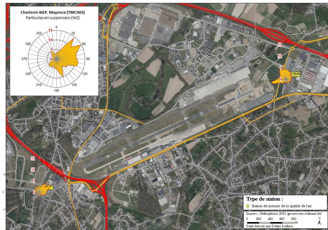
Figure 6.3.4 : Monoxyde d'azote (NO) – Roses de pollution – (01/01/2024 au 30/06/2024)
