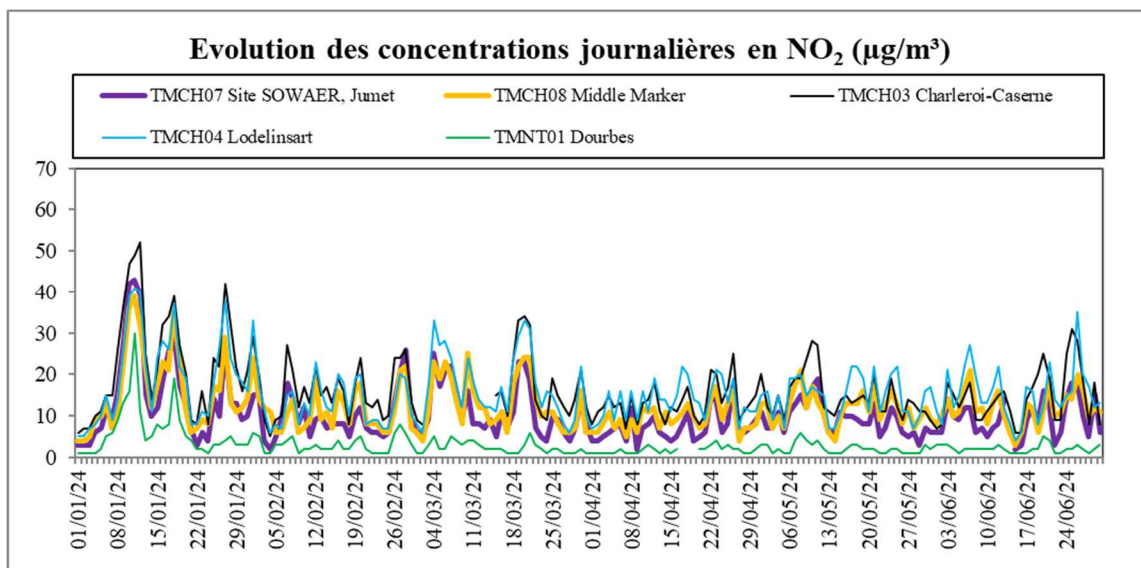
Figure 6.5.1 : Dioxyde d'azote (NO 2 ) – Evolution des concentrations journalières – (01/01/2024 au 30/06/2024)
