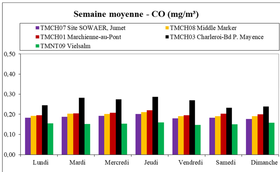
Figure 5.3.3 : Monoxyde de carbone (CO) - Semaine moyenne - (01/01/2024 au 30/06/2024)
