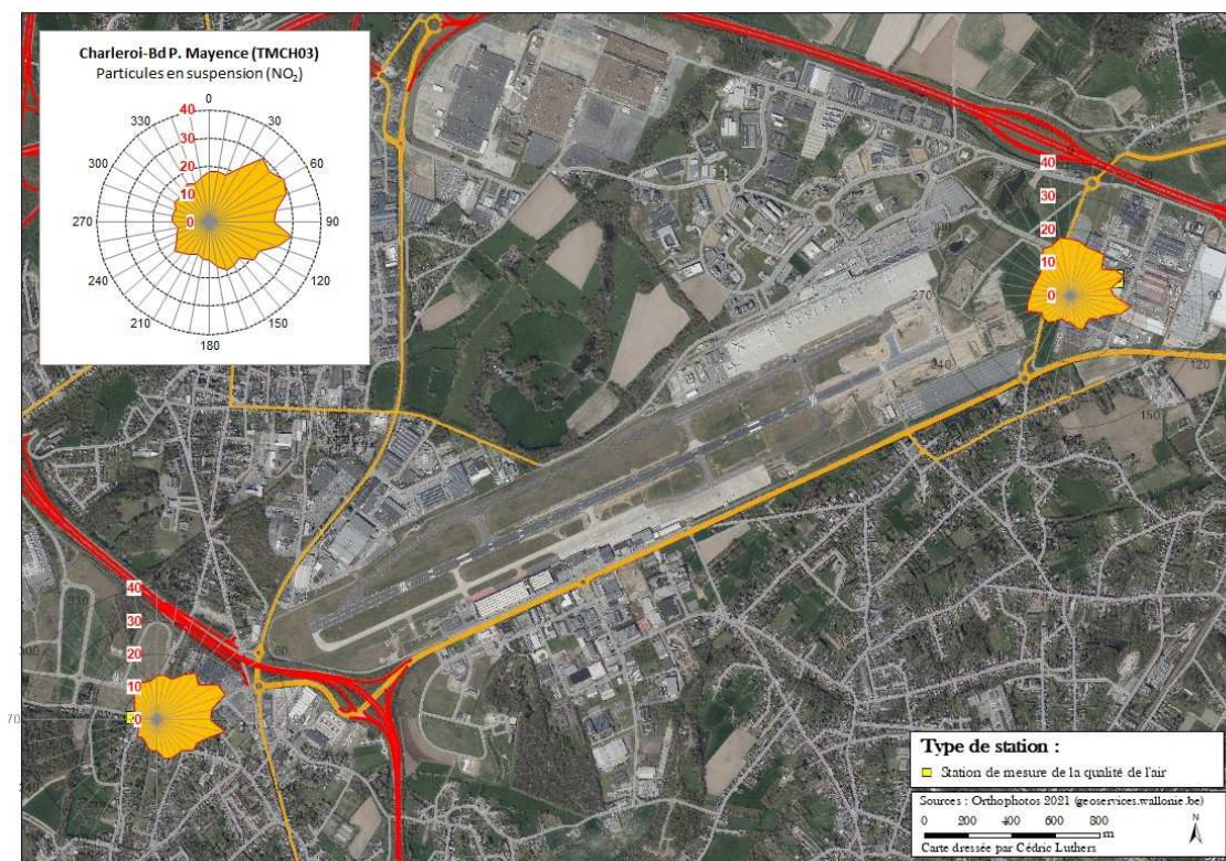
Figure 6.5.4 : Dioxyde d'azote (NO 2 ) – Roses de pollution – (01/01/2024 au 30/06/2024)
