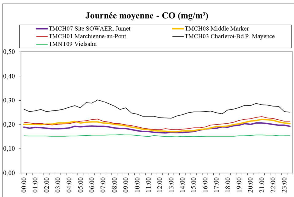
Figure 5.3.2 : Monoxyde de carbone (CO) - Journée moyenne - (01/01/2024 au 30/06/2024)
