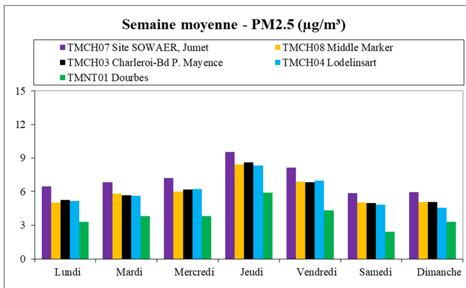
Figure 4.5.3 : PM2.5 – Semaine moyenne – (01/01/2024 au 30/06/2024)
