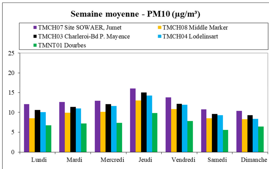
Figure 4.3.3 : PM10 – Semaine moyenne – (01/01/2024 au 30/06/2024)
