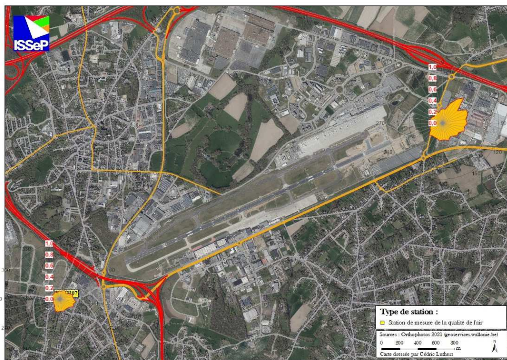
Figure 7.3.2 : Benzène ( C_6H_6 ) – Roses de pollution – (01/01/2024 au 30/06/2024)
