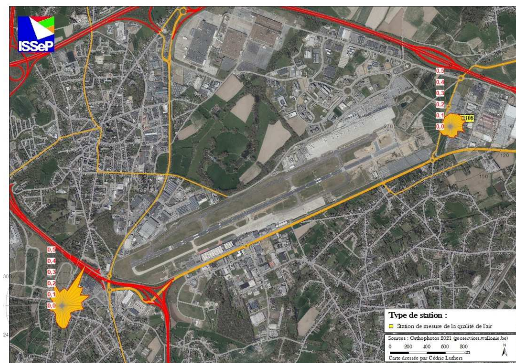
Figure 7.3.5 : m+p-xylènes ( C_8H_{10} ) – Roses de pollution – (01/01/2024 au 30/06/2024)
