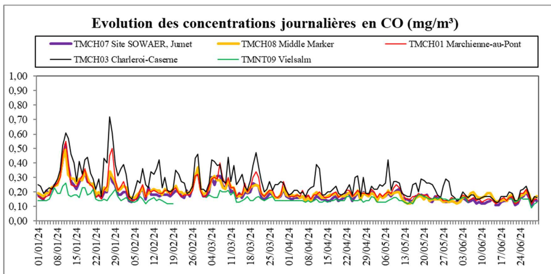
Figure 5.3.1 : Monoxyde de carbone (CO) – Evolution des concentrations journalières – (01/01/2024 au 30/06/2024)
