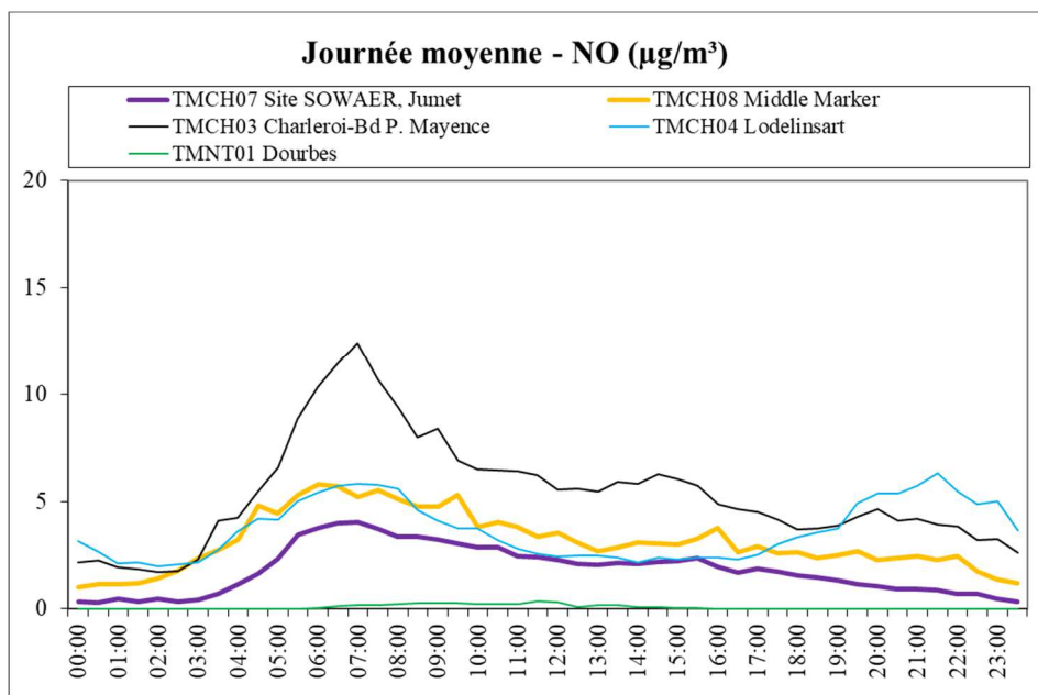
Figure 6.3.2 : Monoxyde d'azote (NO) – Journée moyenne – (01/01/2024 au 30/06/2024)
