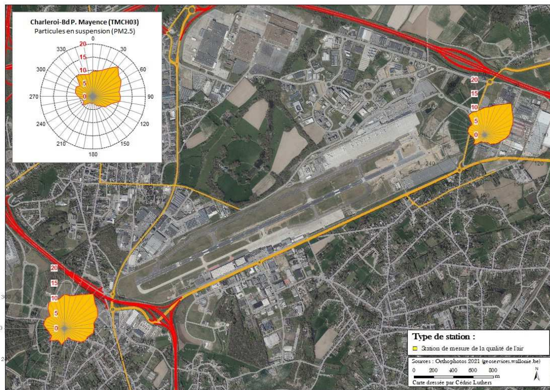
Figure 4.5.4 : PM2.5 – Roses de pollution – (01/01/2024 au 30/06/2024)
