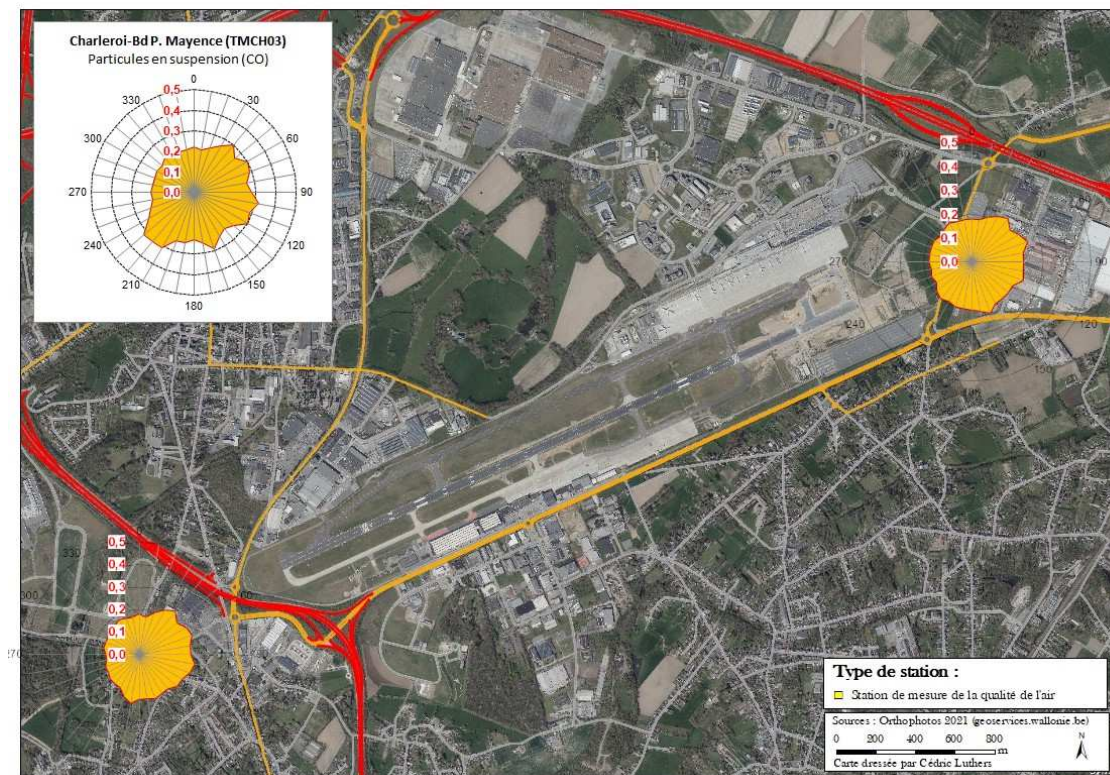
Figure 5.3.4 : Monoxyde de carbone (CO) - Roses de pollution - (01/01/2024 au 30/06/2024)
