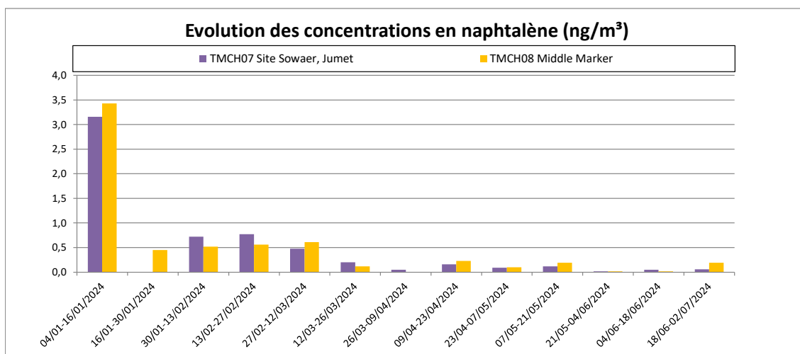
Figure 8.3.1 : Naphtalène (C 10 H 8 ) – Evolution des concentrations – (04/01/2024 au 02/07/2024)
